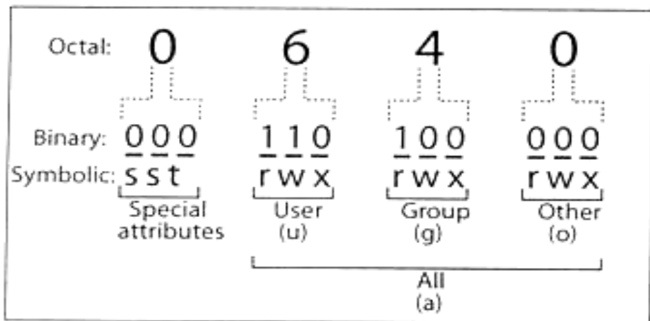
Рис. 3. Значение битов в правах на файл
